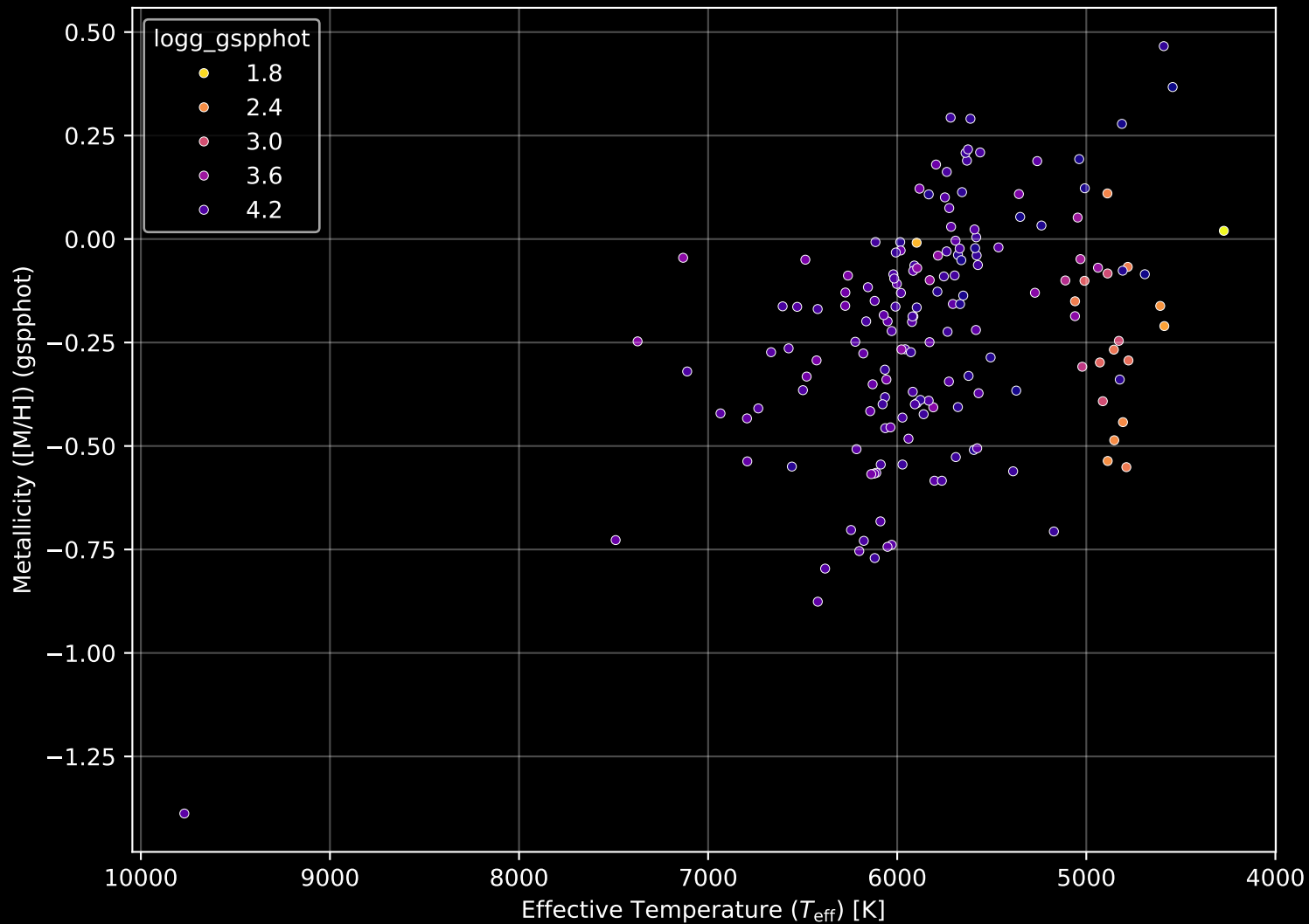
GALAH DR4 Field: [7215] Stellar Population Parameters (n= 167)
