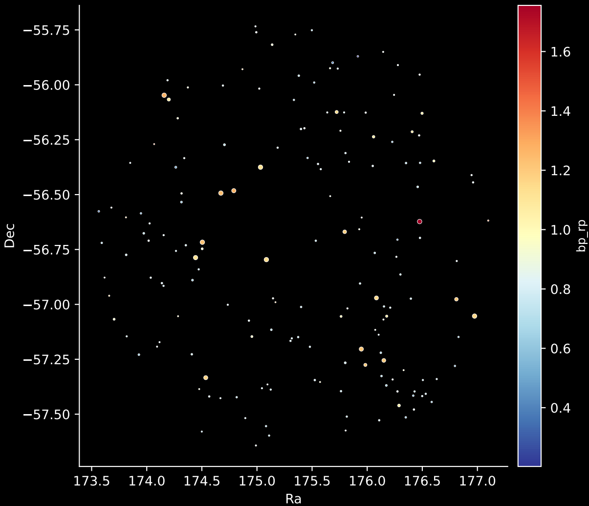
GALAH DR4 Field: [7215] Stars: 167
